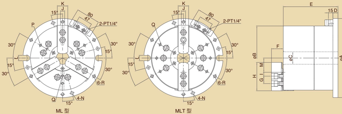
寸法図 ≫ Dimensions
