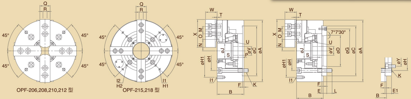
寸法図 > Dimensions
